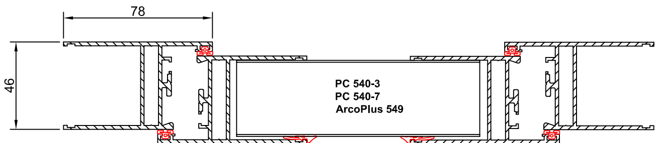
Schnitt B - B
